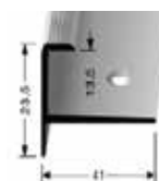
HARO Treppenkantenprofil 812 EB SBS Art. Nr. 88626812_
