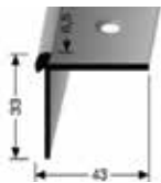
HARO Treppenkantenprofil 874 EB SBS Art. Nr. 88626874_
