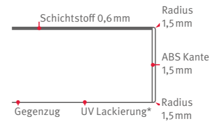
Modell 100 / 1,5
