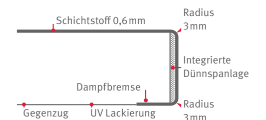
Modell 300 / 3
