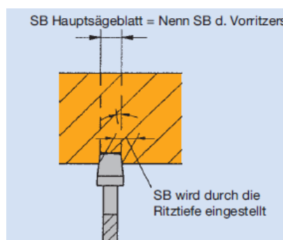
Einsatzschema konisches Ritzkreissägeblatt. Bei der Instandsetzung der Werkzeuge (immer Satzweise) müssen die Schnittbreiten einander abgestimmt werden
