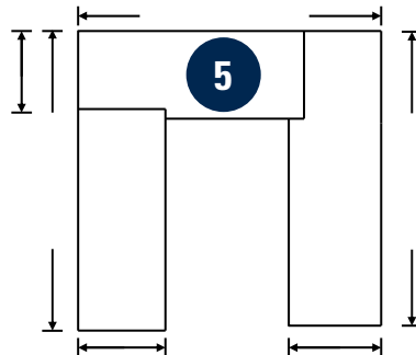
Eck-Verbindung für L- oder U-Form
